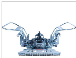
Hydrauliczny chwytak Probst HVZ-UNI-II
