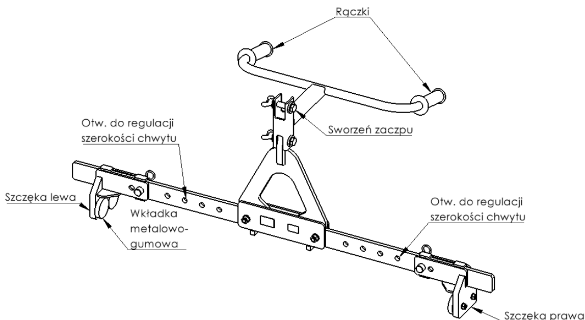
Rys.1 Objaśnienie elementów ustawczych narzędzia
