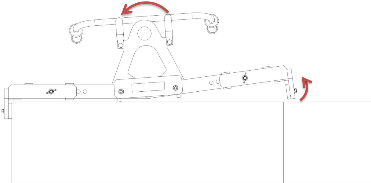
Rys.1 Wypięcie chwytnika z przenoszonego elementu.
