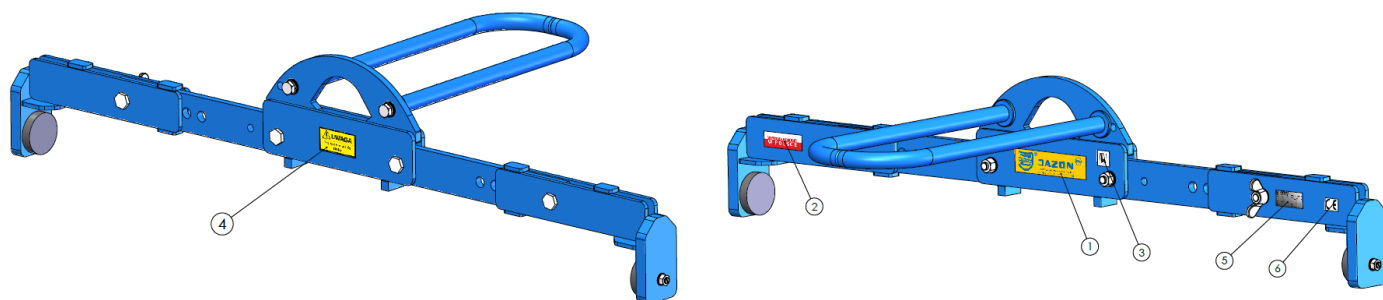
Rys. Rozmieszczenie tabliczek informacyjno-ostrzegawczych
